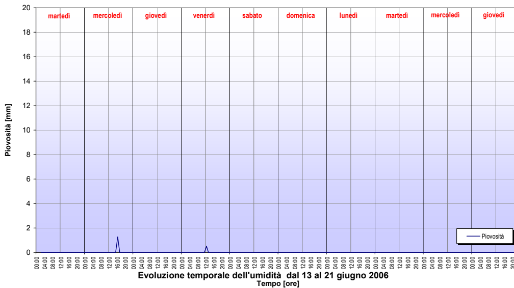
Evoluzione temporale della piovosità dal 13 al 21 giugno 2006
