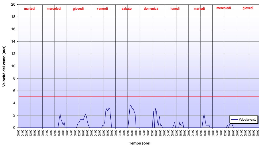
Evoluzione temporale della velocità del vento dal 13 al 21 giugno 2006
